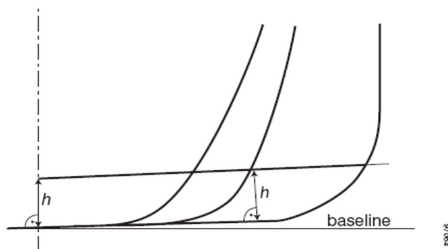
Obrázok 1 - Hraničné línie palivovej nádrže
