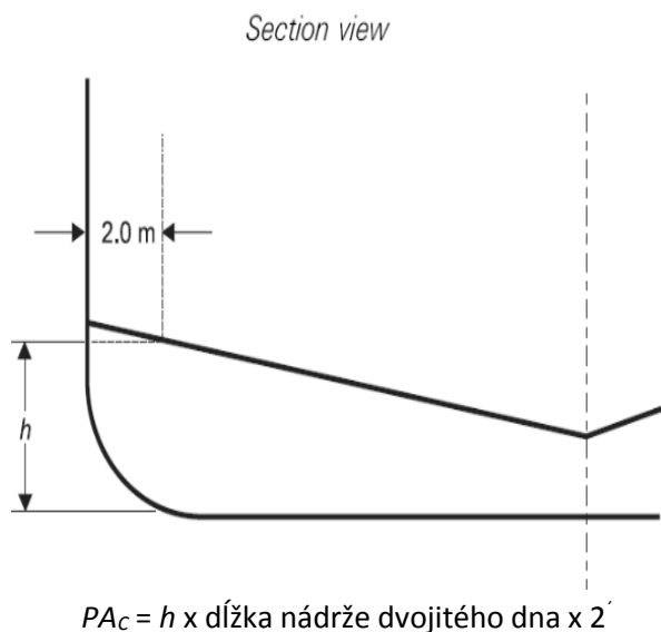
Obrázok 8 – Meranie h pre výpočet PA_C nádrží dvojitého dna so šikmými hornými plochami (2)
